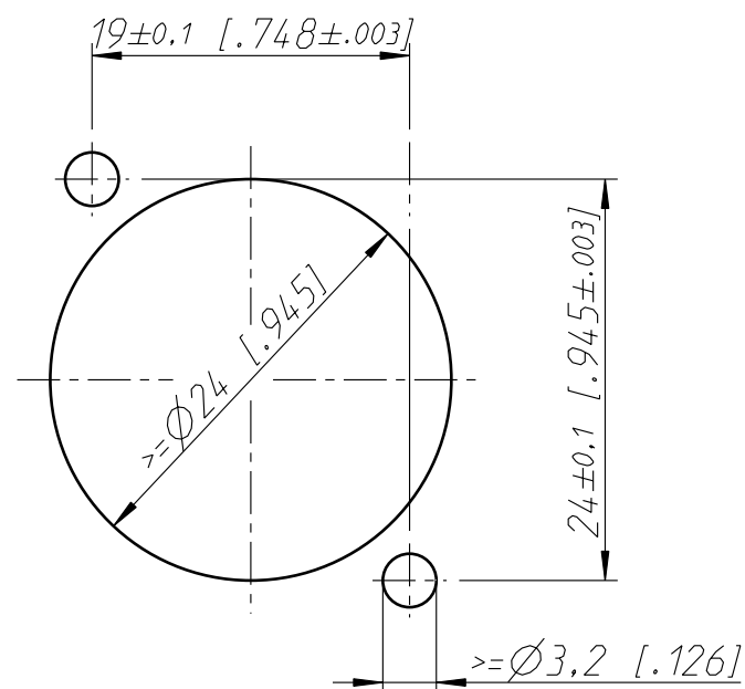
Frontplattenausschnitt (Rückseite) Panel Cutout (rear side)
