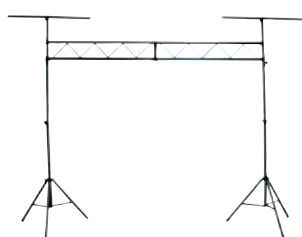
Enkelvoudig lichtstatief met lier - Max. last: 60kg - Materiaal: aluminium - Ø balken: 35mm - Afmetingen: 1,5 tot 2,5m (max.) x 1.2m breed - Gewicht: 15kg
